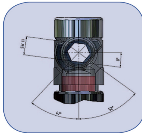
Befestigung 2351 fitting 2351
